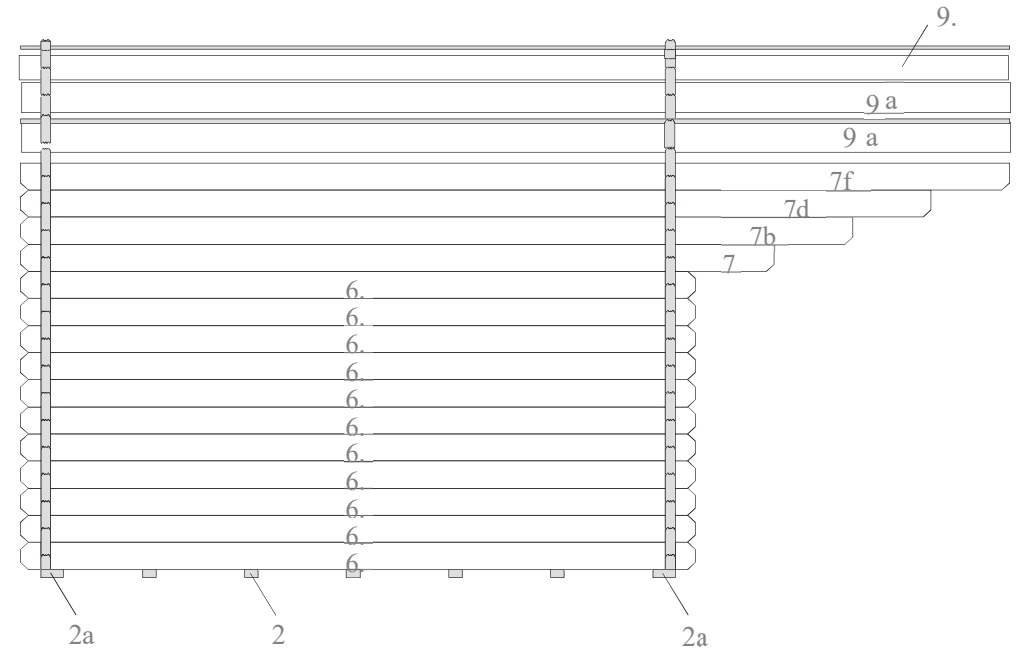
VORDERWAND
