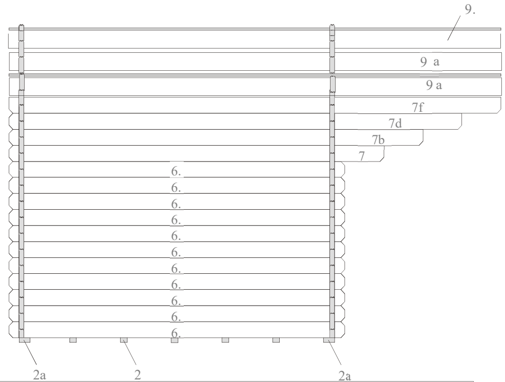
VORDERWAND
