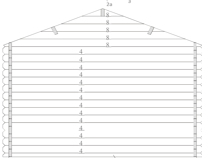
HINTERWAND
